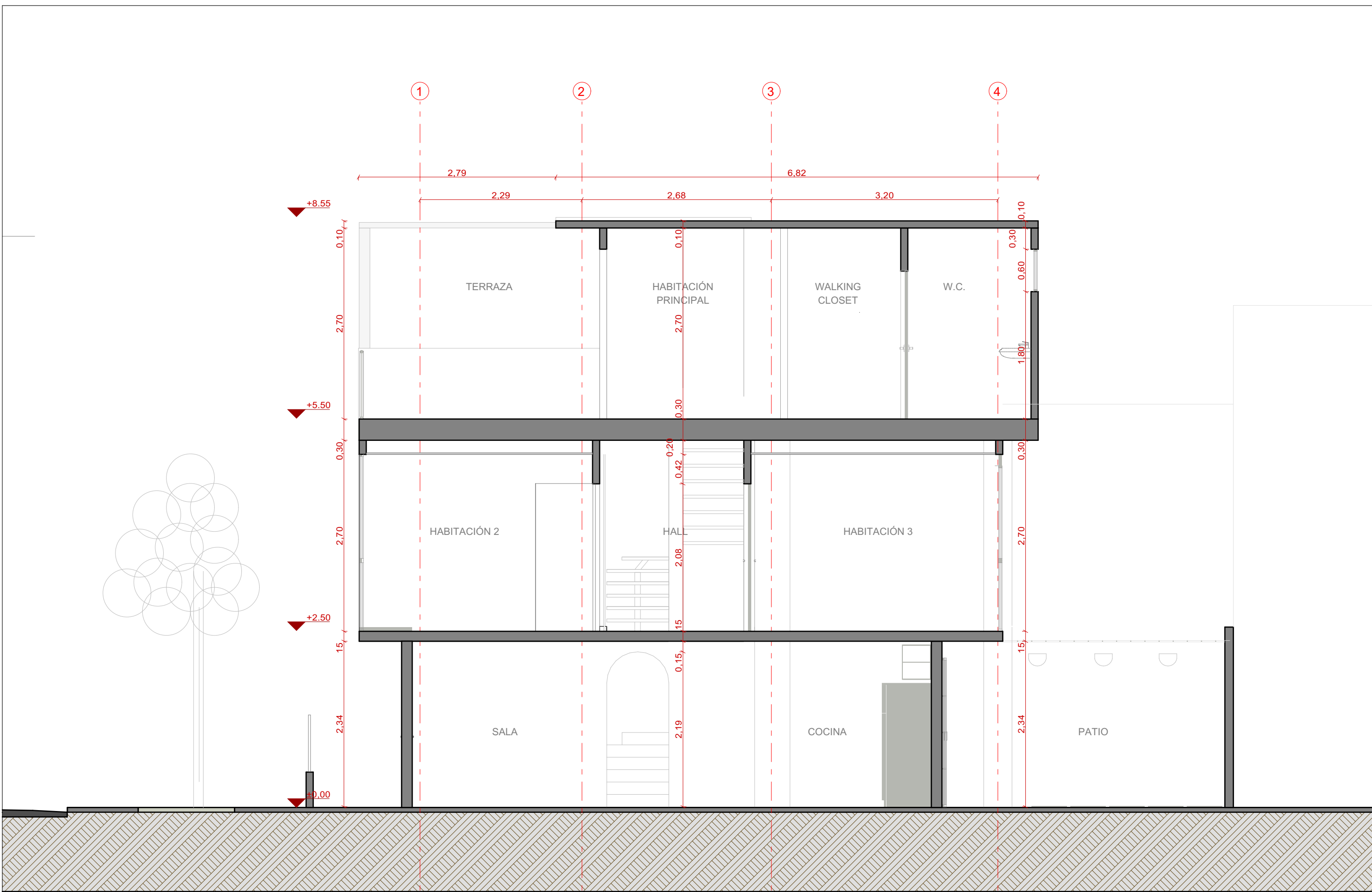
Corte B-B'
