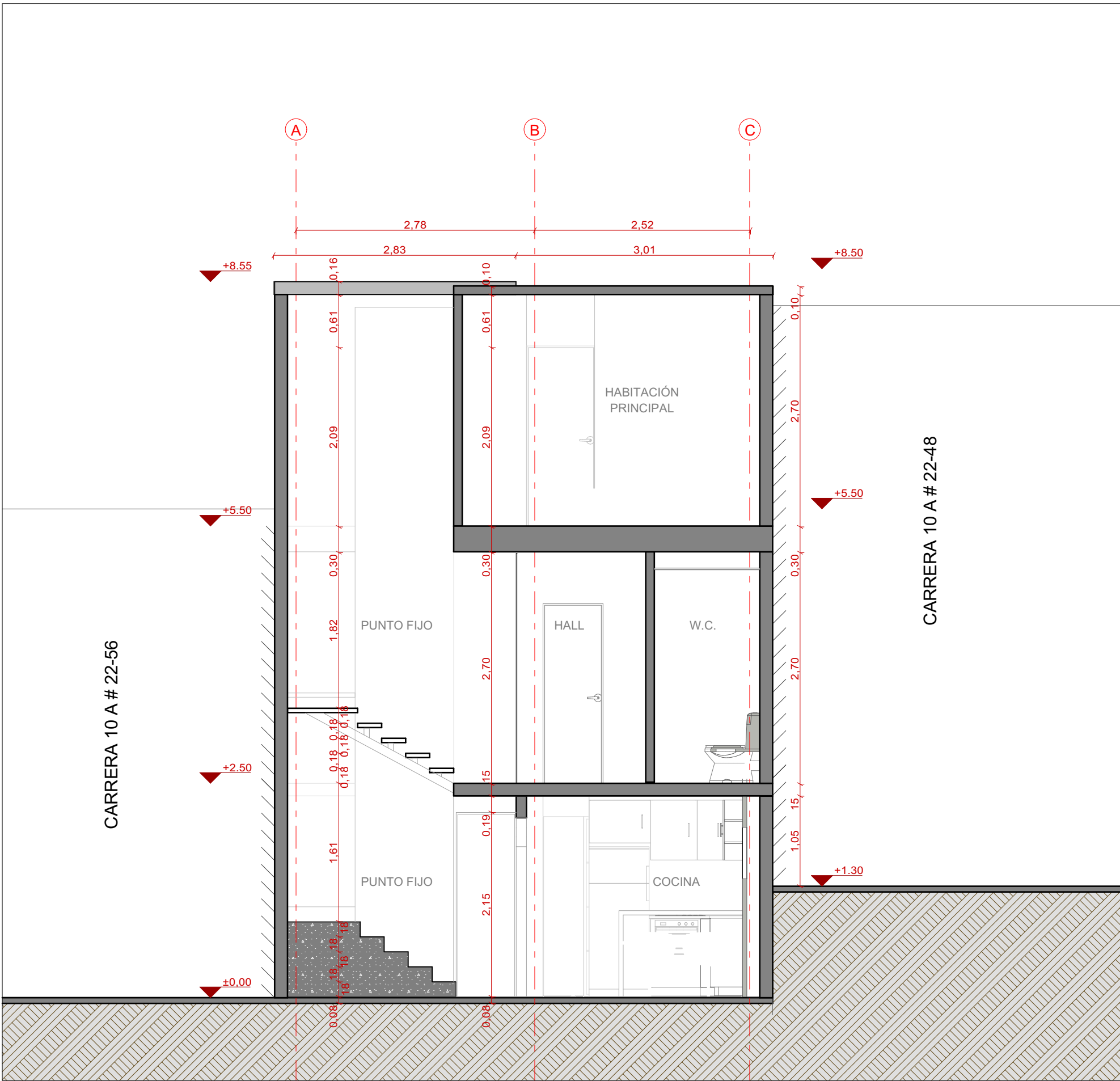
Corte A-A'
